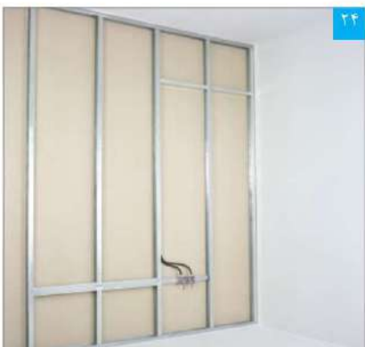
درزهای افقی به صورت خمیرچین نسبت به یکدیگر قرار می‌گیرند (به محل سازه‌های پشت بند توجه شود)
